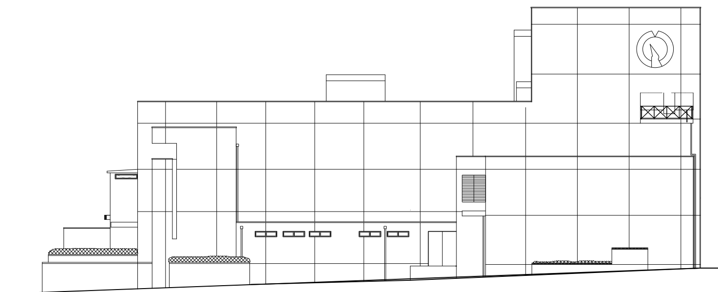
南側立面図
