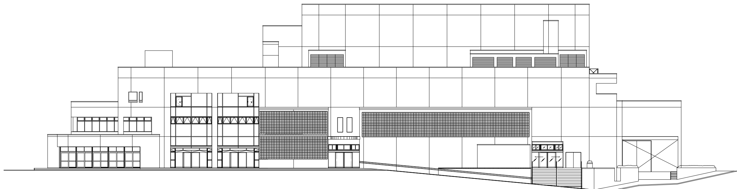
西側立面図
