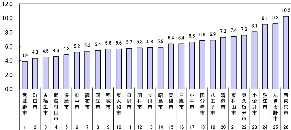
2-11. グラフ 公債費比率 (単位: %)
