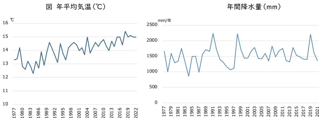
出典:気象庁 HP データ(青梅気象台)
