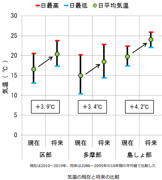
図 気温の現在と将来の比較
